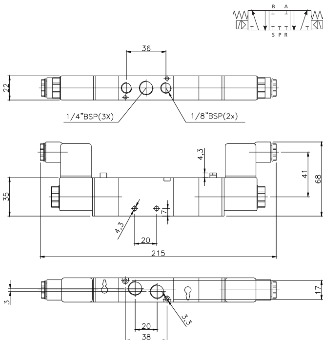
Solenóide Autocentrante - 5V - CFE _____ VC3699
